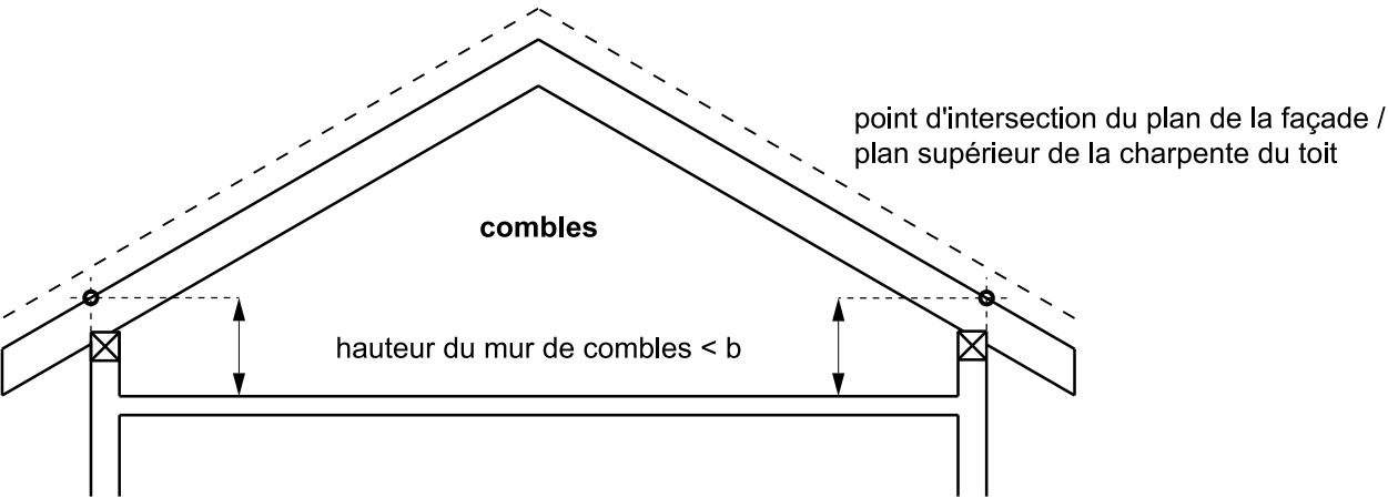
b hauteur du mur de comble admise
